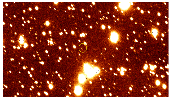
11/20 国立天文台すばる望遠鏡で撮影された「はやぶさ 2」撮影時の地球から「はやぶさ 2」までの距離は約 580 万 km。写真中央の○内。(国立天文台ホームページより)
